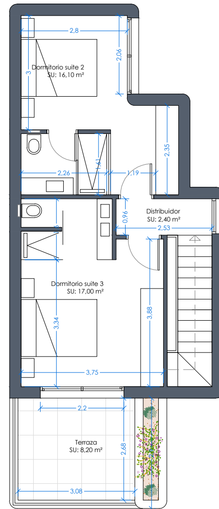
PLANTA PRIMERA
